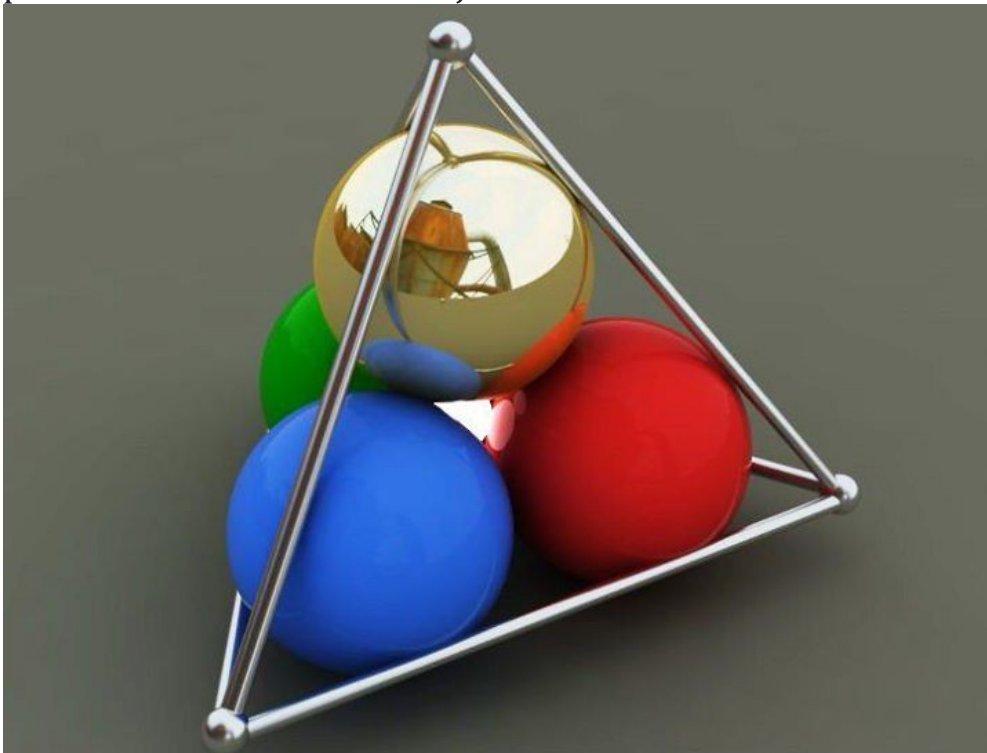
A Tetraéder a 4 gömbbel,
